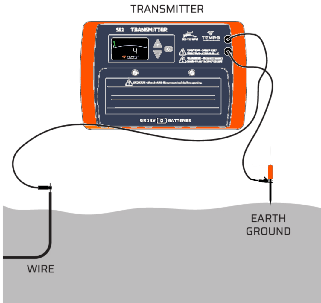
図1 送信機の直接接続（金属に接続）
