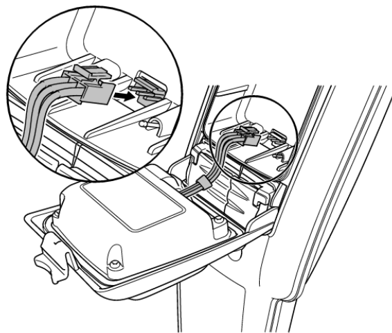
図 4.7 リチウムイオンリード線の接続
