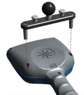
図12.14: ブラケットの位置決め
