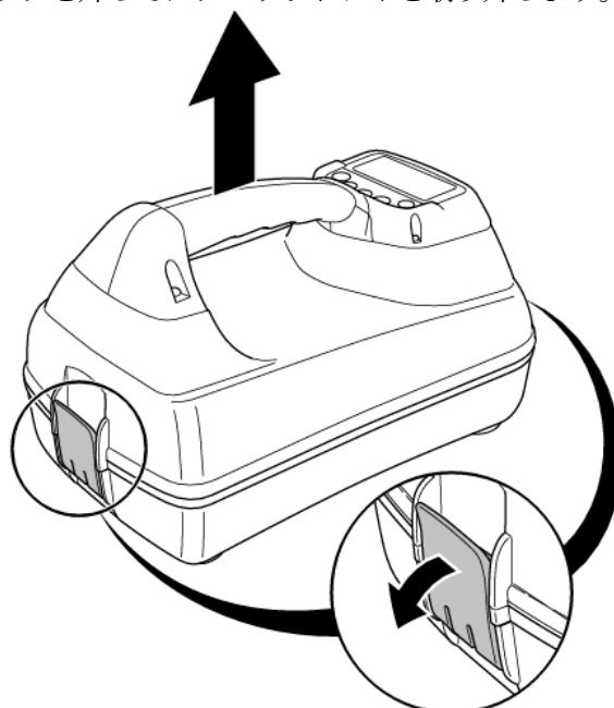
図 4.8 ラッチを外してアクセサリトレイを取り外します
