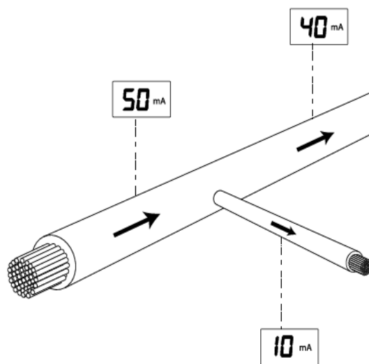
図 6.3 電流測定値
