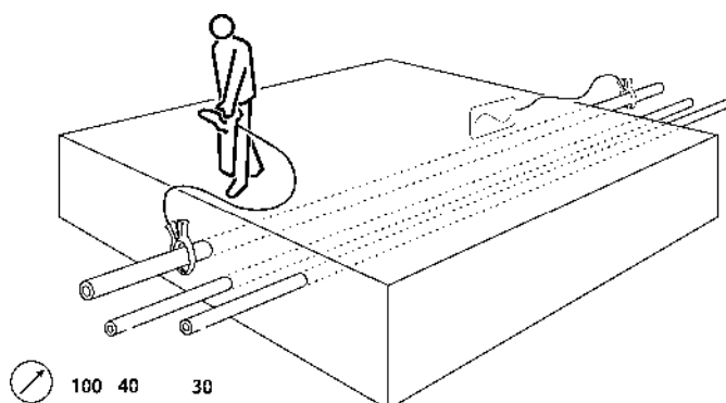
図 12.1: クランプの接続
